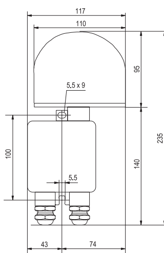
CEL-32-48-F dimensions
