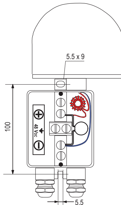
CEL-32-48-F terminal box
